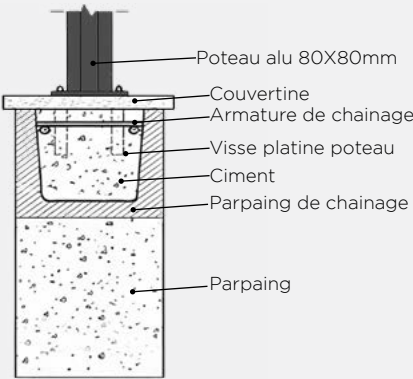
Schéma de chaînage obligatoire
